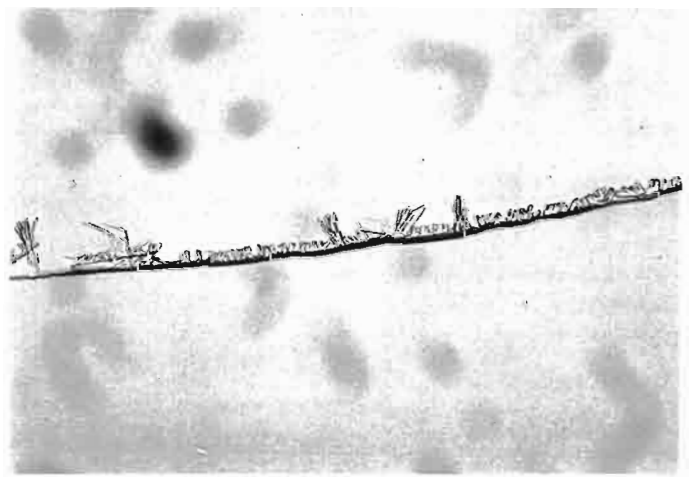
5 Links Mitte Gipskristalle ( \text{CaSO}_4 \cdot 2\text{H}_2\text{O} ) beim Nachweis von Calcium mittels Zugabe von 1 M Schwefelsäure. Bildbreite = 1,4 mm
