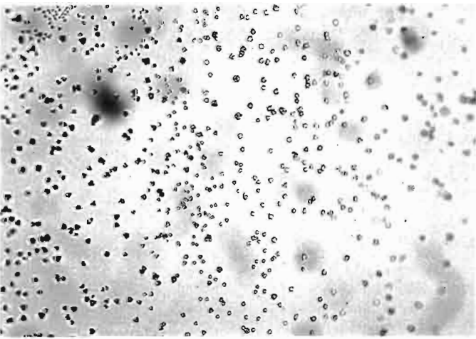
3 Links oben Natrium-Wismuth-Sulfat-Kristalle. Bildbreite = 1,4 mm
