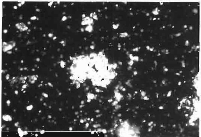
1 Zwei Beispiele für Gipskristalle unter gekreuzten Polarisatoren in Streupräparaten (siehe Text).
